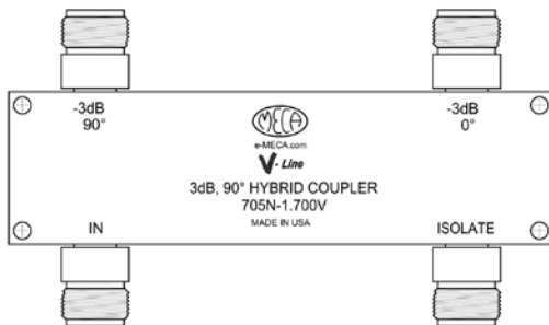
705N-1.700V
